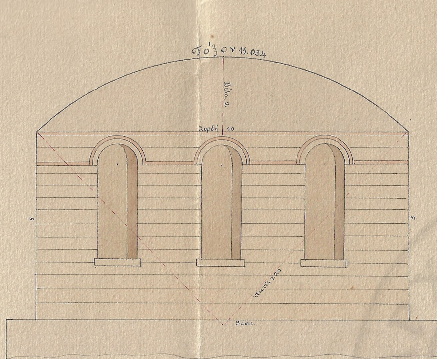
Voute Surbaissée. Θόλος Βραχυτενής.
